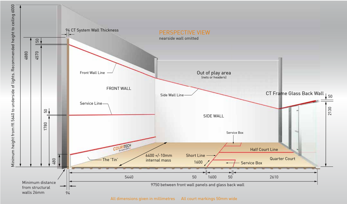
Требуемые размеры для кортов со стенами CT System
